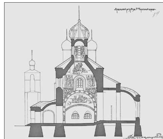
Рис. 4. Поперечный разрез Глазово-Тярлевской церкви. РГИА. Ф. 854. Оп. 1. Д. 67. Л. 35
