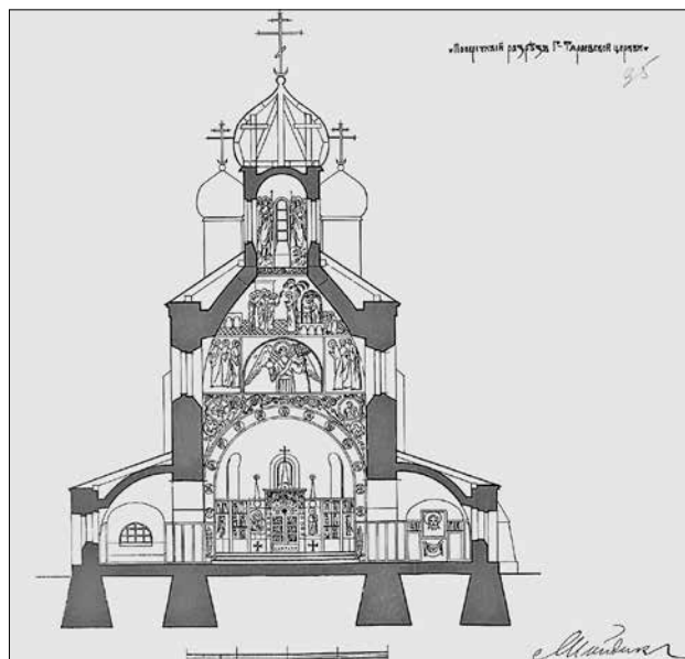
Рис. 3. Продольный разрез Глазово-Тярлевской церкви. РГИА. Ф. 854. Оп. 1. Д. 67. Л. 34
